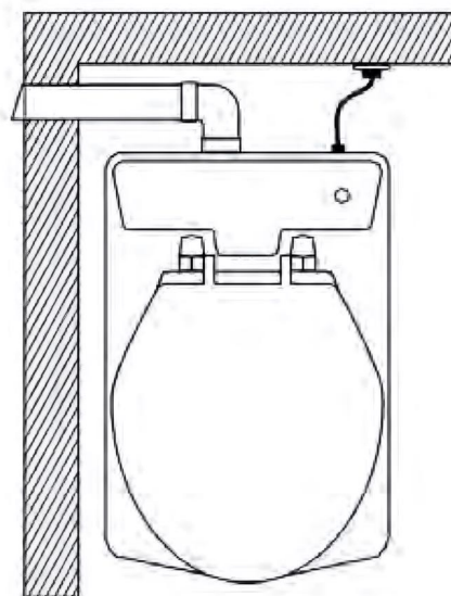
DET ÄR OCKSÅ MÖJLIGT ATT VINKLA RÖRET FÖR ATT SEDAN GÅ UT GENOM YTTERVÄGG
