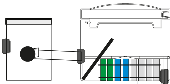
Parallellkopplade BioBox M för att fördubbla kapaciteten Sedd från sidan och ovanifrån med en fördelningsbrunn
